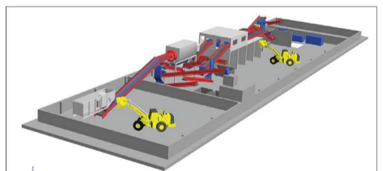
Mechaninio rūšiavimo įrenginiai pastato viduje
